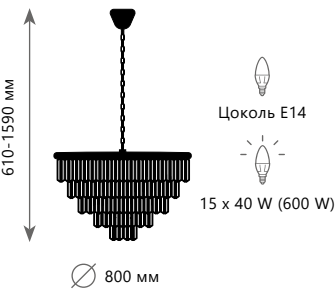
Подвесная люстра A 10019/800C ● ⊘ металл, хрусталь ● золото, прозрачный
