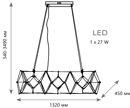
Подвесной светильник A 10257/1320 ● ▨ металл ● хром 1890 Lm | 3000 K
