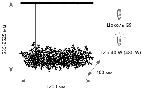
Подвесной светильник A 10101/4 CHROME ● ⊘ металл ● хром
