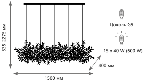
Подвесной светильник A 10101/5 GOLD ● ⊘ металл ● золото
