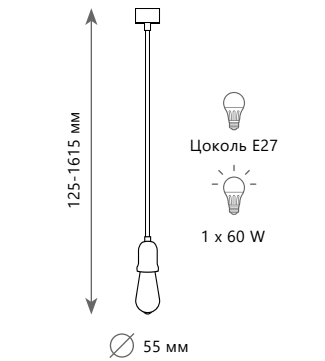
Подвесной светильник A 10091 ● ● металл, полимерная смола ● белый
