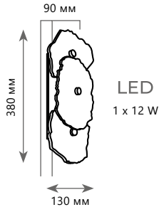
Настенный светильник A 10248/3W металл, испанский мрамор медь, мрамор 840 Lm | 3000 K
