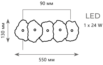
Настенный светильник A 10248/5W металл, испанский мрамор медь, мрамор 1680 Lm | 3000 K
