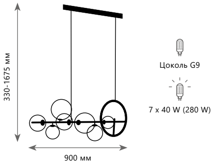
Подвесной светильник A 10023/900 ● ⊘ металл | стекло ● черный | прозрачный
