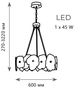
Подвесной светильник A 10248/600 металл, испанский мрамор медь, мрамор 3150 Lm | 3000 K
