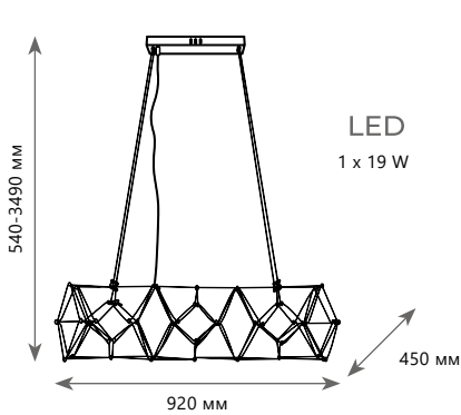
Подвесной светильник A 10257/920 ● ▨ металл ● хром 1330 Lm | 3000 K
