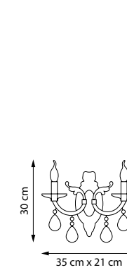
694622 БРА 2 x E14 max 40W 1,8 kg
