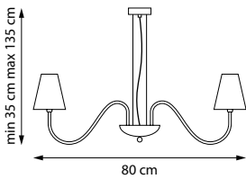
758084 ЛЮСТРА ПОДВЕСНАЯ 8 x G9 max 40W 3 kg
