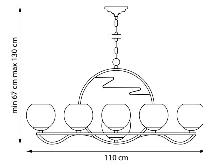
762077 ЛЮСТРА ПОДВЕСНАЯ 7 x E14 max 40W 5,4 kg
