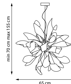
754267 ЛЮСТРА ПОДВЕСНАЯ ■ 754269 ЛЮСТРА ПОДВЕСНАЯ ■ ■ 6 x G9 LED 6W 2,3 kg
