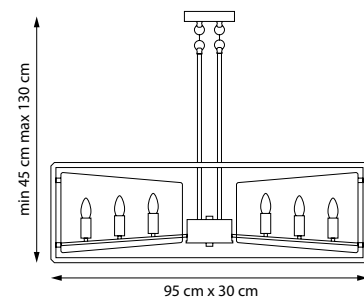
713327 ЛЮСТРА НА ШТАНГЕ 12 x E14 max 40W 5 kg
