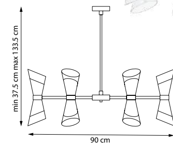
817167 ЛЮСТРА НА ШТАНГЕ 16 x E14 max 40W 10,9 kg
