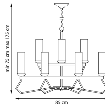
723085 ЛЮСТРА ПОДВЕСНАЯ 8 x E14 max 40W 6,4 kg
