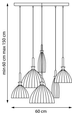
810160 ЛЮСТРА ПОДВЕСНАЯ 6 x E14 max 40W 9 kg
