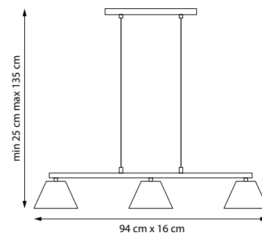
719223 ЛЮСТРА ПОДВЕСНАЯ 2 x GX53 max LED 12W 1 kg
