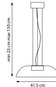
809061 3000K ● ЛЮСТРА ПОТОЛОЧНАЯ LED 12W 3000K 600LM 2,4 kg
