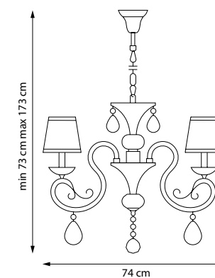
693082 ЛЮСТРА ПОДВЕСНАЯ 8 x E14 max 40W 11,2 kg
