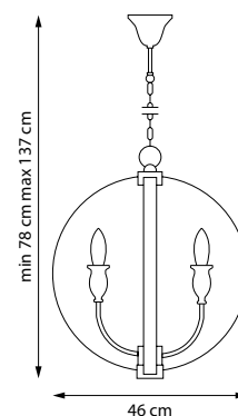
731067 ЛЮСТРА ПОДВЕСНАЯ 6 x E14 max 40W 5,6 kg
