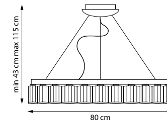
812126 ЛЮСТРА ПОДВЕСНАЯ ■ □ 12 x G9 LED 6W 5 kg
