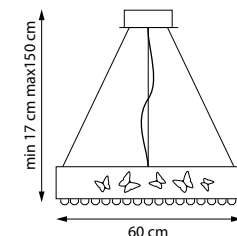
701101 3000K ● ПОДВЕС LED 10W 3000K 757LM 2,4 kg
