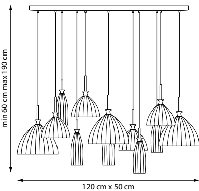
810010 ПОДВЕС 810013 ПОДВЕС 1 x E14 max 40W 1,1 kg
