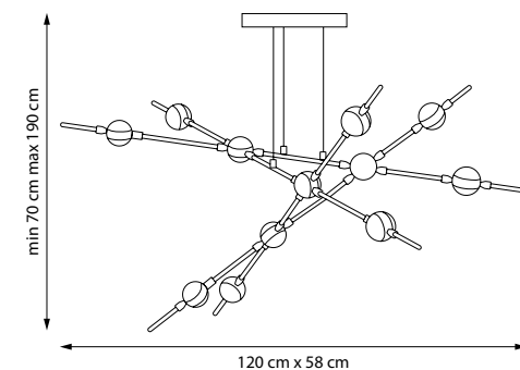
745147 ЛЮСТРА ПОТОЛОЧНАЯ LED 50W 4000K 4000Lm 2,7 kg
