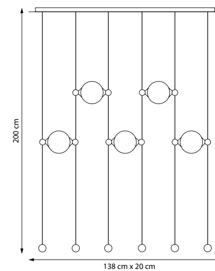
815501 3000 ● ЛЮСТРА ПОДВЕСНАЯ 5 x LED 8,5W 3000K 8 kg
