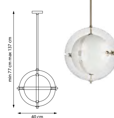
816043 ЛЮСТРА НА ШТАНГЕ 8 x G9 max 40W 7,4 kg
