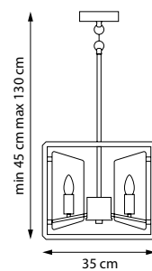
713037 ЛЮСТРА НА ШТАНГЕ 3 x G9 max 40W 4,5 kg
