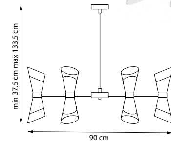
817164 ЛЮСТРА НА ШТАНГЕ 16 x E14 max 40W 10,9 kg
