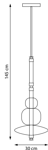
737540 3000K ● ЛЮСТРА НА ШТАНГЕ LED 24W 3000K 1200LM 6,15 kg
