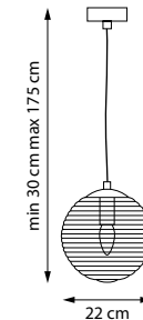
803115 ПОДВЕС 1 x E27 max 40W 0,9 kg
