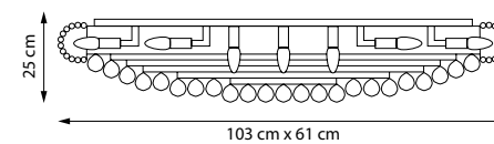
704174 ЛЮСТРА ПОТОЛОЧНАЯ 17 x E14 max 40W 19 kg
