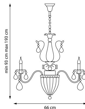
790114 ЛЮСТРА ПОДВЕСНАЯ 8 x E14 max 60W 3 x E14 max 60W 12,7 kg
