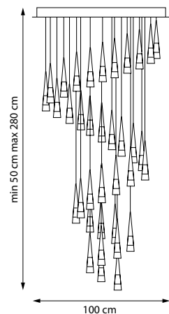
757361 3000K ● ЛЮСТРА ПОДВЕСНАЯ LED 180W 3000K 9000LM 22,5 kg
