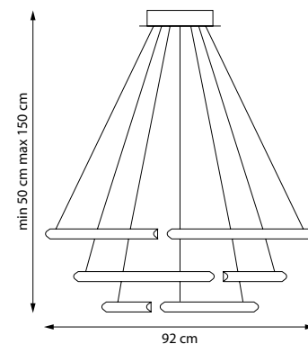
814223 3000 ● ЛЮСТРА ПОДВЕСНАЯ LED 58W 3000K 2900Lm 3,4 kg
