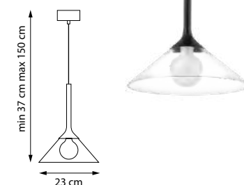
801203 ПОДВЕС 1 x G9 max 6W 0,7 kg
