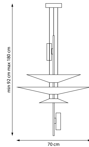
814532 3000K ● ПОДВЕС LED 18W 3000K 560LM 4,7 kg
