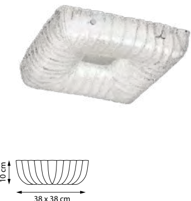
820440 ЛЮСТРА ПОТОЛОЧНАЯ 4 x E14 max 60W 7,9 kg
