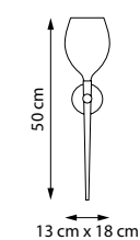
807610 БРА 1 x E14 max 40W 1,7 kg
