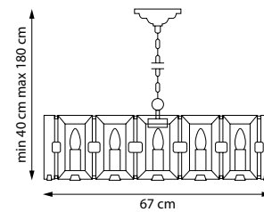
713267 ЛЮСТРА ПОДВЕСНАЯ ■ □ 6 x E14 max 40W 8,6 kg
