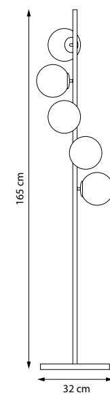
815753 ТОРШЕР 815757 ТОРШЕР 5 x E14 max 40W 7,5 kg
