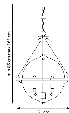
816037 ЛЮСТРА НА ШТАНГЕ 3 x E27 max 40W 3,4 kg
