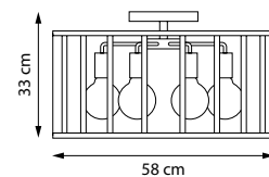
798251 ЛЮСТРА ПОТОЛОЧНАЯ 5 x E27 max 40W 4,6 kg
