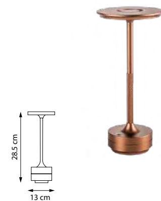
745901 3000K ● / 4000K ○ / 6000K ● НАСТОЛЬНАЯ ЛАМПА LED 2W 3000/4000/6000K 170LM 0,6 kg
