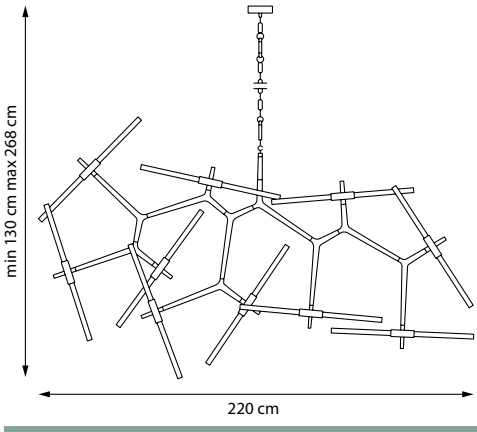
742203 ЛЮСТРА ПОДВЕСНАЯ 20 x G9 LED 6W 8,5 kg
