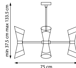
817012 ПОДВЕС 817014 ПОДВЕС 1 x E14 max 40W 1 kg
