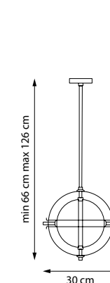
816033 ЛЮСТРА НА ШТАНГЕ 4 x G9 max 40W 3,1 kg
