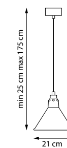
765027 ПОДВЕС 1 x E14 max 40W 0,5 kg
