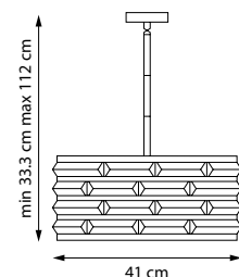
746068 ЛЮСТРА НА ШТАНГЕ 6 x E14 max 40W 5,6 kg
