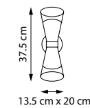
817622 БРА 817624 БРА 817627 БРА 2 x E14 max 40W 1,2 kg
