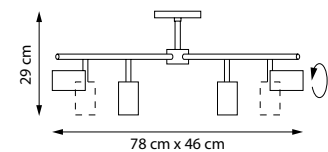
LR728378 ЛЮСТРА ПОТОЛОЧНАЯ
