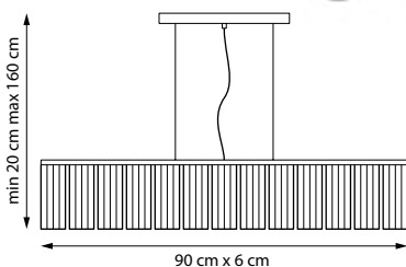
718263 ЛЮСТРА НА ШТАНГЕ
