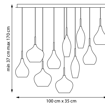
803120 ЛЮСТРА ПОДВЕСНАЯ 12 x E14 max 40W 11,9 kg
