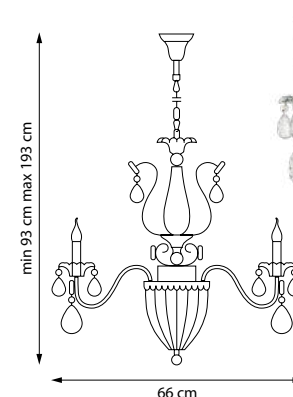
790112 ЛЮСТРА ПОДВЕСНАЯ 8 x E14 max 60W 3 x E14 max 60W 12,7 kg
