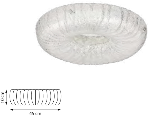
820360 ЛЮСТРА ПОТОЛОЧНАЯ 6 x E14 max 60W 9 kg
