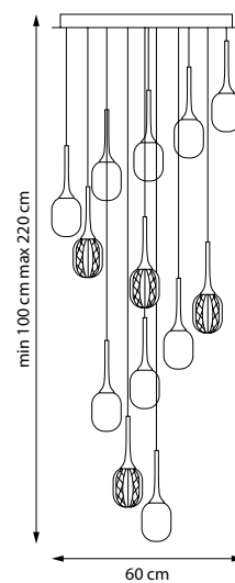
738073 3000K ● ПОДВЕС LED 7W 3000K 578LM 0,7 kg
